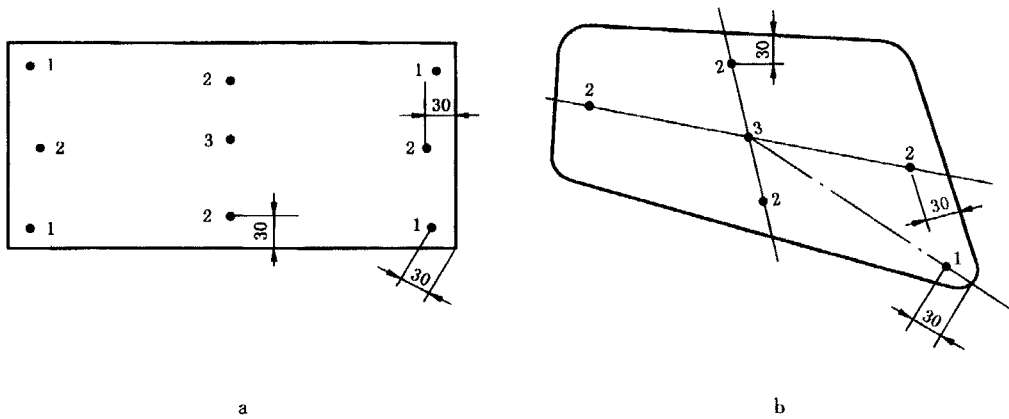
图 2 平型或单曲面试样冲击点位置
