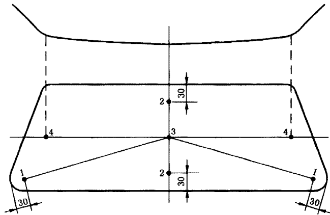
图 3 复合曲面试样冲击点位置
