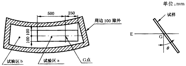
风窗玻璃在实车安装角下的投影图
